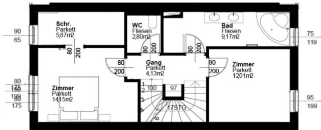
OG
