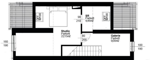
DG
