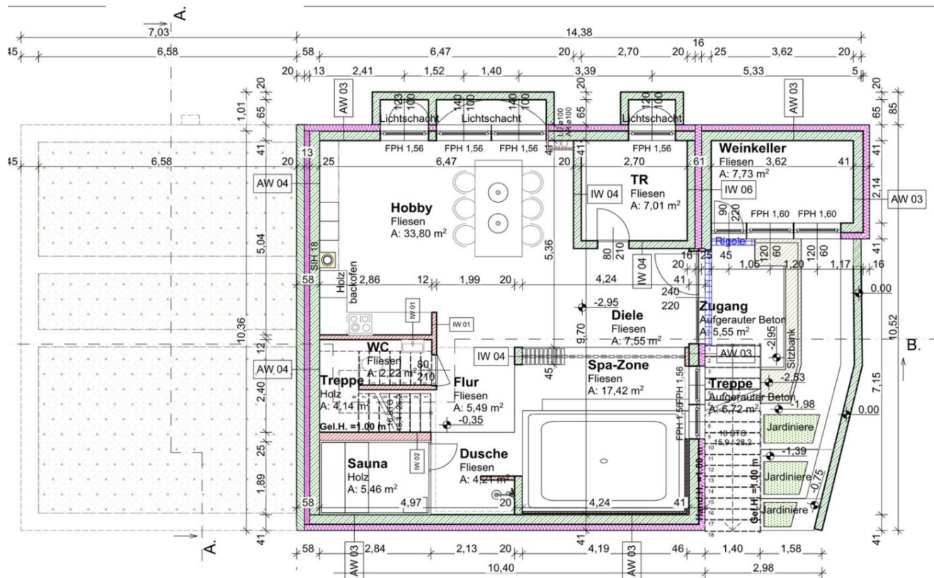
Grundriss Kellergeschoss
