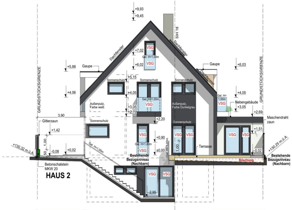
Ost-Ansicht
