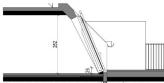
Schnitt 47.B
