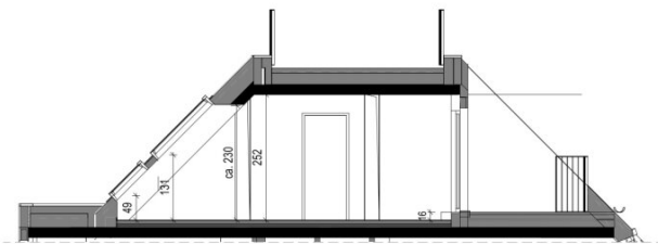
Schnitt 39.B
