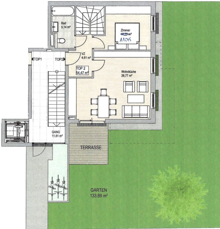
GRUNDRISS ERDGESCHOSS 1/100
