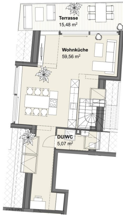
1. DACHGESCHOSS | TOP 6 | M 1:100
