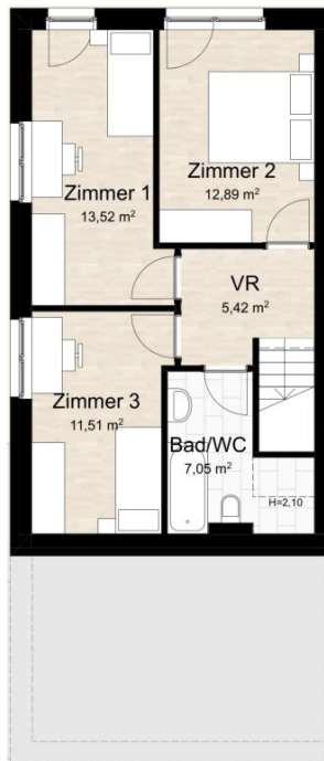
Haus 05 - Urscha 203a Ebene 0 Maßstab 1:100
