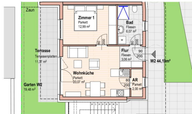
WOHNUNG 2 ERDGESCHOSS
