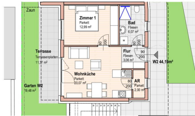
WOHNUNG 2 ERDGESCHOSS
