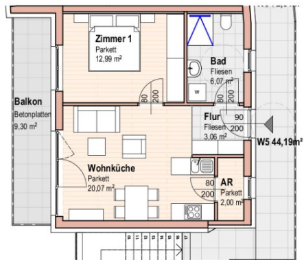
WOHNUNG 5 OBERGESCHOSS
