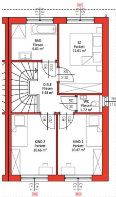
OBERGESCHOSS M 1:100
