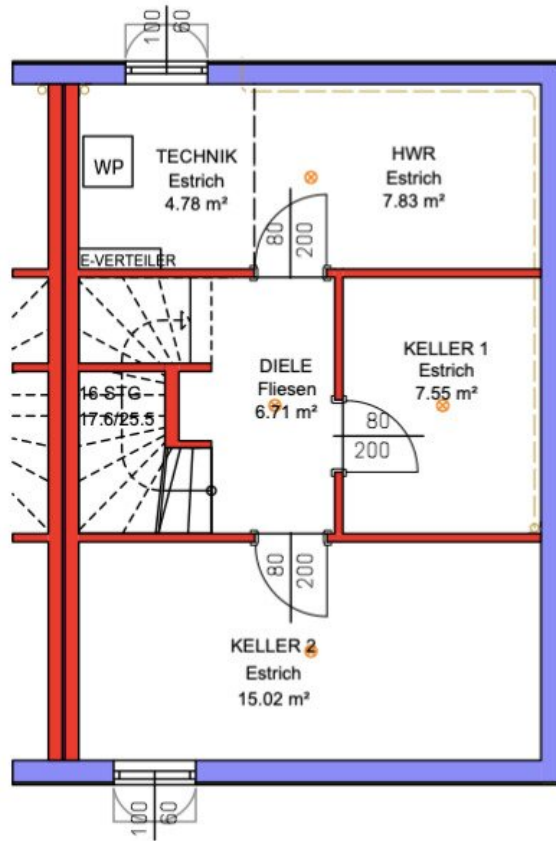
KELLERGESCHOSS M 1:100
