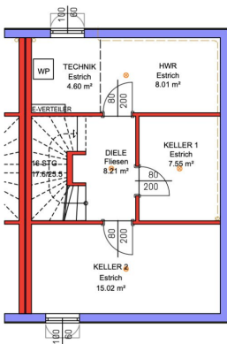
KELLERGESCHOSS M 1:100
