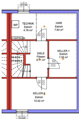
KELLERGESCHOSS M 1:100
