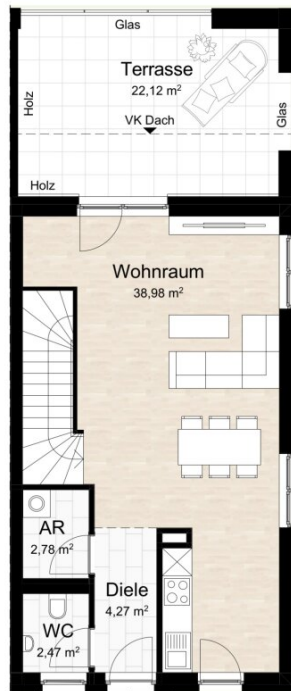
Haus 12 - Urscha 206b Ebene 1 Maßstab 1:100
