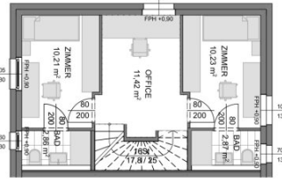
Obergeschoß
