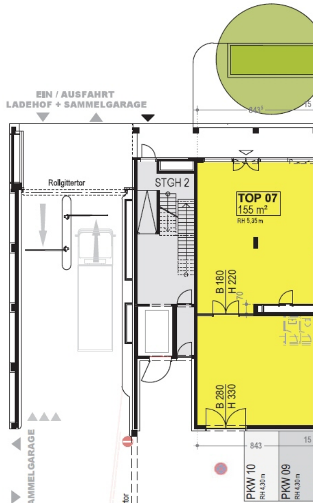
Top07_Grundrisspläne
