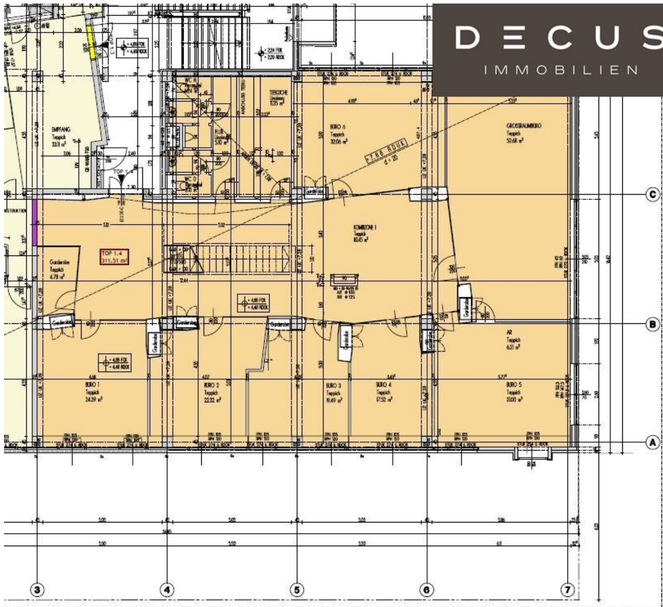
1. OBERGESCHOSS
