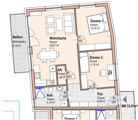
WOHNUNG 6 OBERGESCHOSS
