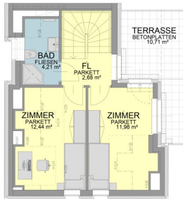
1 OBERGESCHOSS
