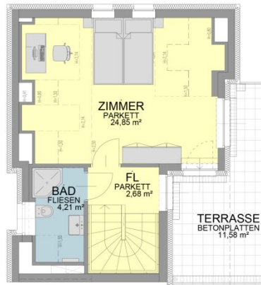
DACHGESCHOSS
