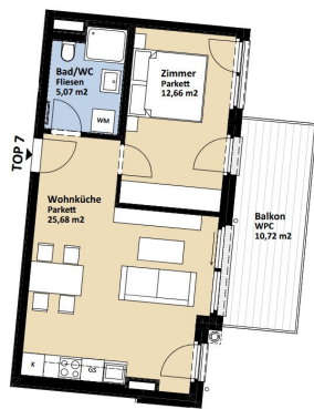
Grundriss TOP 7 Obergeschoß 1:100
