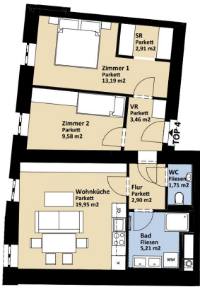
Grundriss TOP 4 Erdgeschoß 1:100
