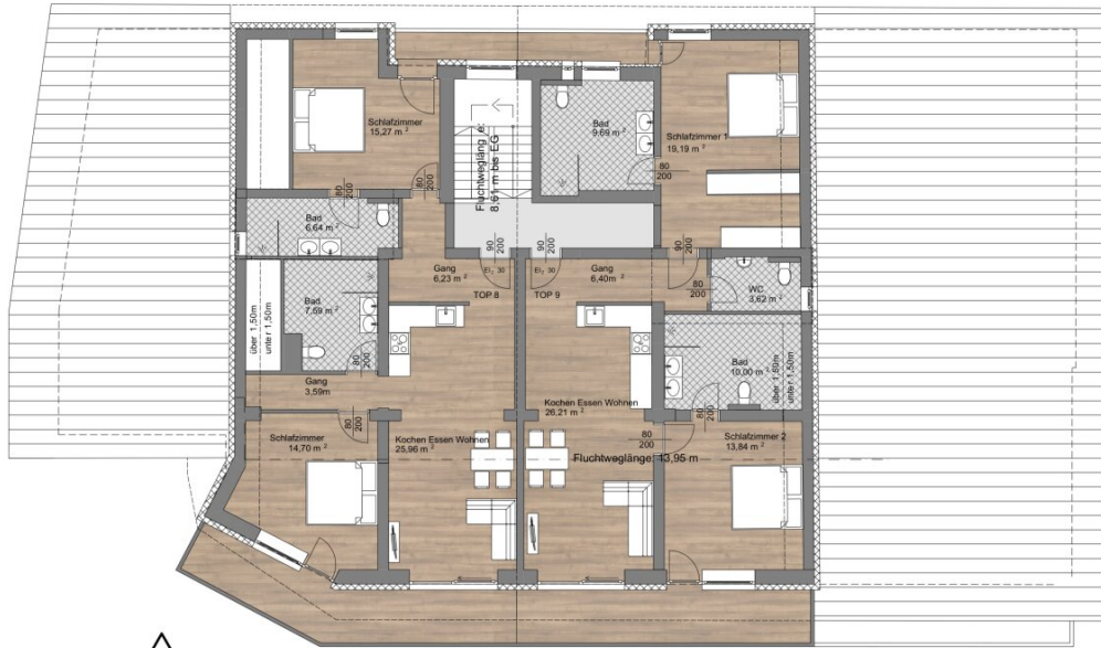
Dachgeschoss
