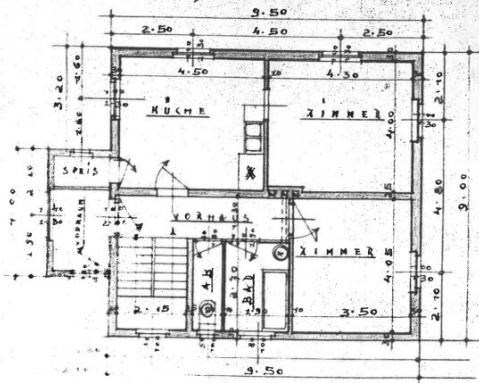
PARTERREGUNDRISS
