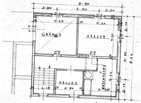
HELLERGRUNDRISS
