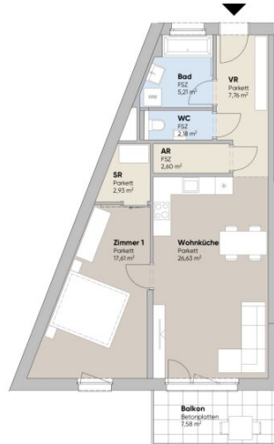
1. Obergeschoß
