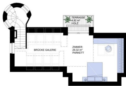
2. DACHGESCHOSS
